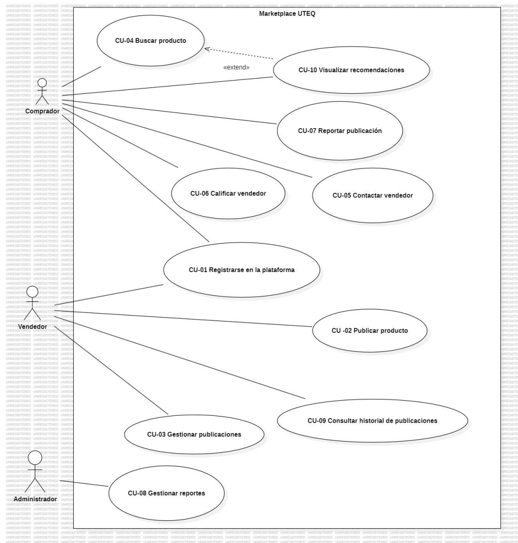
Figura 1 Diagrama de Casos de Uso del sistema Marketplace UTEQ
